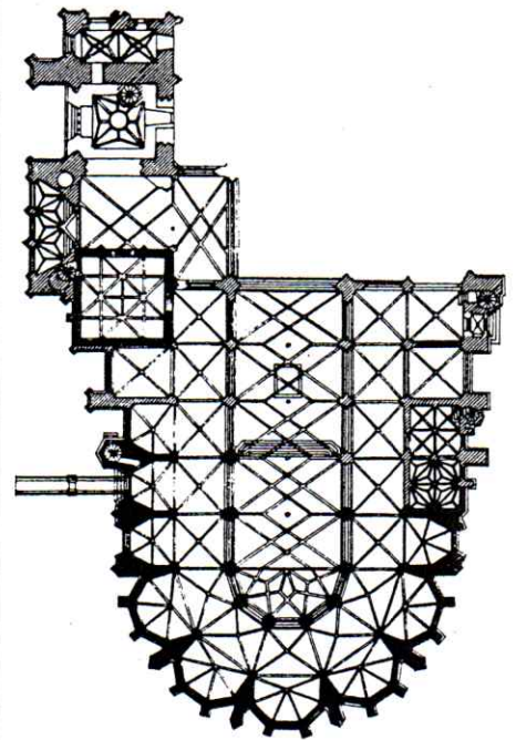
Půdorys Svatovítské katedrály do r. 1419. Podíl Matyáše z Arrasu je znázorněn černě, Parléřova huť — šrafovaně.
